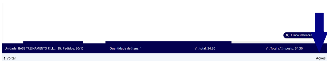
Figura 7: Botão Ações
